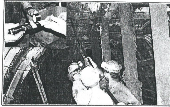
NABÍJENÍ ROZNĚTNÉ NÁLOŽKY DO STROPU CHODBY
