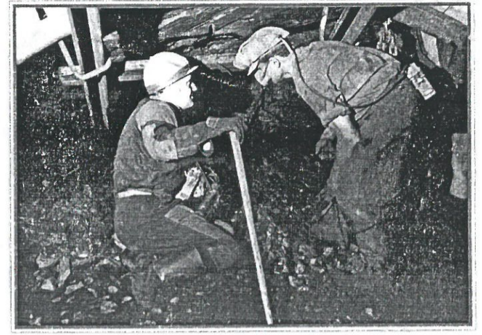
VEDOUČÍ ZÁVODU ČSM-JIH ING. ZDENĚK DOMBROVSKÝ PŘI KONTROLE ČELBY PO TRHACÍ PRÁCI (PO DDPAU)
