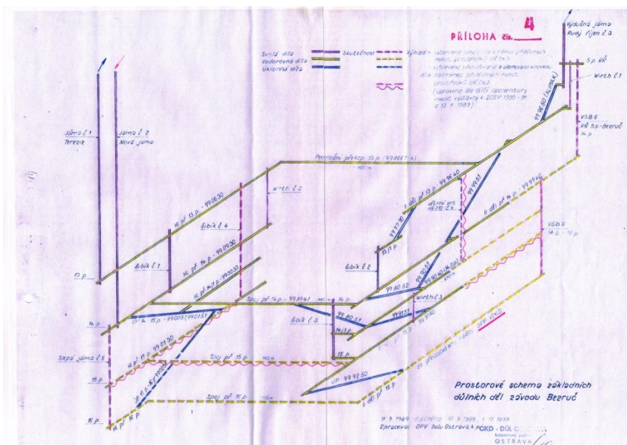
Prostorové schéma důlních děl Dolu Petr Bezruč. / 1969/
