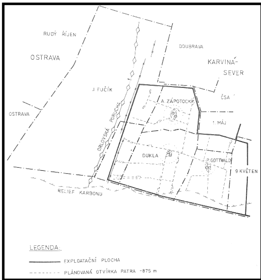
Obr. č. 2 – Otvírka na patře -875 m
